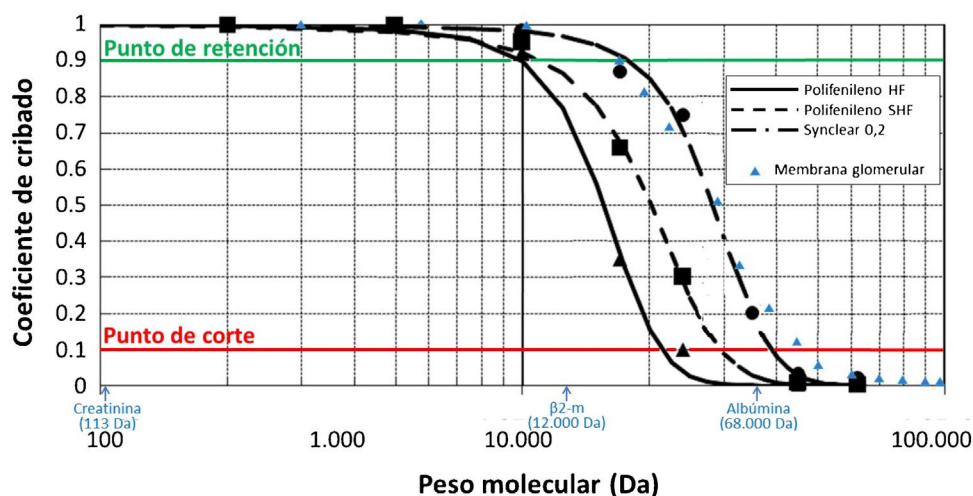
Figura 2 – Representación esquemática de las curvas de cribado de las distintas membranas utilizadas en HFR (Polifenileno HF, Polifenileno SHF, Synclair 0,2). Los puntos de la curva en los que el coeficiente de cribado es de 0,1 y 0,9 para un determinado peso molecular determinan en cada membrana el punto de corte («cut-off») y el punto de retención («retention onset»), respectivamente. Mientras que el punto de corte refleja el peso molecular a partir del cual el 90% de los solutos va a quedar retenido, el punto de retención señala el peso molecular a partir del cual se va a retener más de un 10% de los solutos. Como puede verse en la gráfica, Synclair 0,2 difiere mucho de Polifenileno HF y SHF tanto en su «retention onset» como en su «cut-off». Esto se traduce en un mayor coeficiente de cribado de la membrana Synclair y, por tanto, en un mayor aclaramiento de sustancias de mediano peso molecular y de toxinas ligadas a proteínas, una vez pasen a través de la resina. Adaptado de: Grandi et al. 40 , Boschetti-de-Fierro et al. 98 y de García-Prieto et al. 99 Los datos referidos a la membrana glomerular (triángulos en azul) se han añadido para su comparación según los datos recogidos por Axelsson et al. 100 β2-m: β2-microglobulina.
