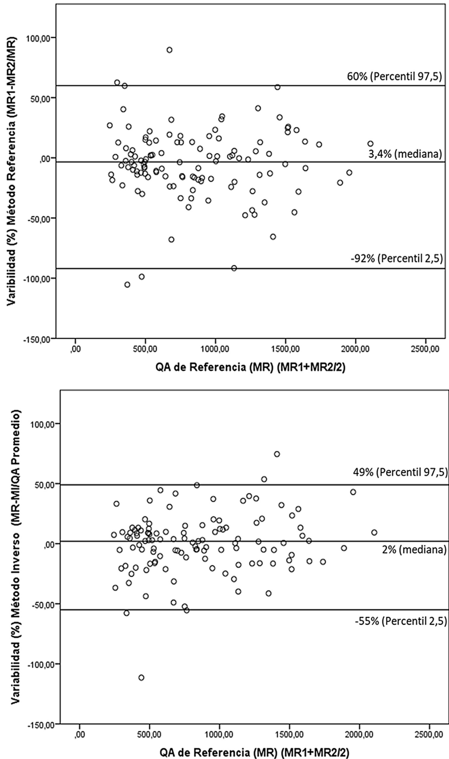
Figura 2 – Representación gráfica según el método de Bland-Altman utilizando el porcentaje de las diferencias entre los valores de Q_A frente el valor medio de las 2 mediciones realizadas con el método de referencia (MR1 + MR2 / 2) , con los correspondientes límites de acuerdo.
